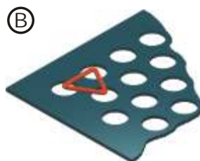
Agujeros redondos tresbolillo 60°
